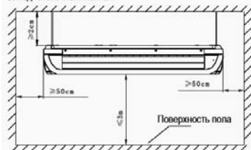
1. Подпотолочный монтаж
