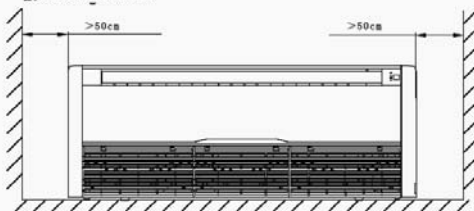
2. Напольный монтаж
